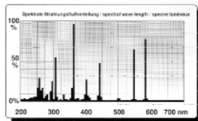
Quecksilberspektrum
